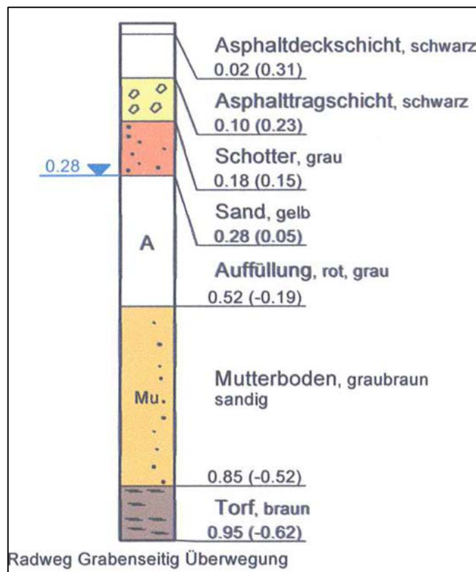
Abb. 1: Bohrprofil (Quelle: Baugrundgutachten Schwitzgebel, April 2018)
